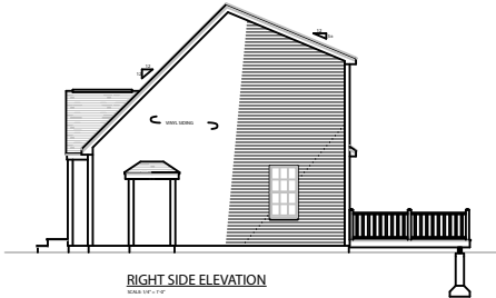
RIGHT SIDE ELEVATION SCALE: 1/8" = 1'-0"
